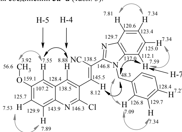
Рис. 1. Отнесение сигналов и эффект Оверхаузера для соединения 3m
