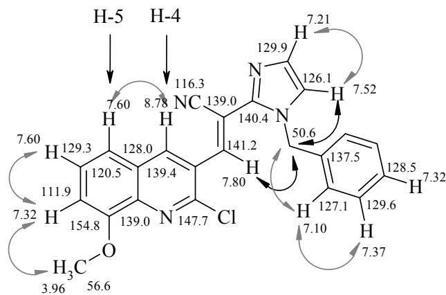
Рис. 3. Отнесение сигналов и эффект Оверхаузера для соединения 7e
