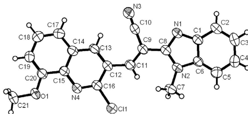
Рис. 2. Молекулярная структура соединения 3i , по данным РСА. Эллипсоиды тепловых колебаний неводородных атомов показаны на уровне 50% вероятности
